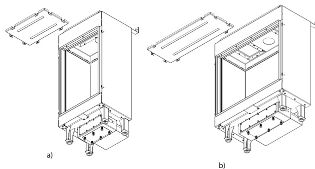
Rys. 12. Demontaż deflektorów: a) LEO45/68, b) LEO76/62 Fig. 12. dismantling the deflectors: a) LEO45/68, b) LEO76/62 Fig. 12. Desmontaje de los deflectores: a) LEO45/68, b) LEO76/62 Obr. 12. Demontáž deflektorů: a) LEO45 / 68, b) LEO76 / 62 Abb. 12. Demontage der Deflektoren: a) LEO45/68, b) LEO76/62 Fig. 12. Smontaggio dei deflettori: a) LEO45/68, b) LEO76/62 Рис 12. Разборка дефлекторов: a) LEO45 / 68, б) LEO76 / 62 Figur 12. Demontering av deflektorer: a) LEO45 / 68, b) LEO76 / 62 Fig. 12. Démontage des déflecteurs : a) LEO45/68, b) LEO76/62 Obr. 12. Demontáž deflektorov: a) LEO45 / 68, b) LEO76 / 62 Kuva 12. Ohjainten purkamisen: a) LEO45 / 68, b) LEO76 / 62 12. ábra A terelőlapok szétszerelése: a) LEO45/68, b) LEO76/62 Fig. 12. Demontering af deflektorer: a) LEO45/68, b) LEO76/62 Фиг. 12. Демонтаж на дефлектори: a) LEO45/68, б) LEO76/62 Slika 12. Demontaža deflektora: a) LEO45/68, b) LEO76/62 Joonis 12. Deflektorite lahtivõtmise: a) LEO45/68, b) LEO76/62 Εικ. 12. Αποσυναρμολόγηση εκτροπέων: α) LEO45/68, β) LEO76/62 Fior 12. Sraonairí a dhíchóimeáil: a) LEO45/68, b) LEO76/62 Rys. 12. Demontaż deflektorów: a) LEO45/68, b) LEO76/62 12. att. Deflektoru demontáža: a) LEO45/68, b) LEO76/62 Fig. 12. Žarmar tad-difletturi: a) LEO45/68, b) LEO76/62 Afb. 12. Demontage van deflektoren: a) LEO45/68, b) LEO76/62 Figura 12. Desmontagem dos defletores: a) LEO45/68, b) LEO76/62 Fig. 12. Demontarea deflectoare: a) LEO45/68, b) LEO76/62 Sl. 12. Demontaža deflektorjev: a) LEO45/68, b) LEO76/62 Fig. 12. Demontering av deflektorer: a) LEO45/68, b) LEO76/62
