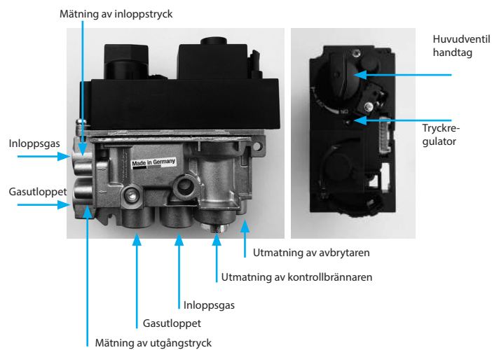
Figur 20. GV60 förare i basläge
