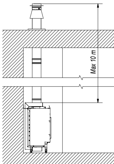
Rys. 9. Wyprowadzenia koncentrycznego systemu kominowego przez dach Fig. 9. The alignment of a concentric chimney system through the roof Fig. 9. La alineación de un sistema de chimeneas concéntrico a través del techo Obr. 9. Vedení koncentrického komínového systému přes střechnu Abb. 9: Die Ausrichtung eines konzentrischen Schornsteinsystems durch das Dach Fig. 9. L'allineamento di un sistema di camini concentrici attraverso il tetto Рис 9. Вывод коаксиальной системы дымохода через крышу Figur 9. Utgang koaksial skorstein systemet gjennom taket Fig. 9 : L'alignement d'un système de cheminée concentrique à travers le toit Obr. 9. Vývody koncentrického komínového systému cez strechu Kuva 9. Samankesken savupiippujärjestelmän ulostulot katon läpi 9. ábra. Koncentrikus kéményrendszer kivezetései a tetőn keresztül Fig. 9. Udgange fra det koncentriske skorstenssystem gennem taget Фиг. 9. Изходи на концентричната коминна система през покрива Slika 9. Izlazi koncentričnog sustava dimnjaka kroz krov
