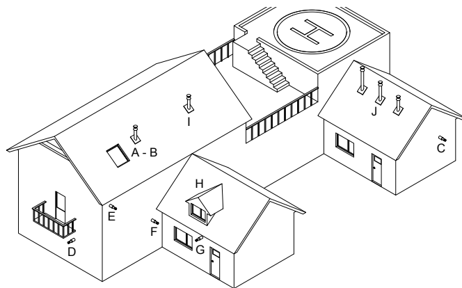
Rys. 7. Możliwe warianty wyprowadzenia koncentrycznego systemu powietrzno- spalnowego dla urządzeń z serii LEO
