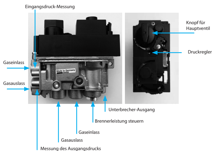
Abb. 20: Regler GV60 in Grundstellung
