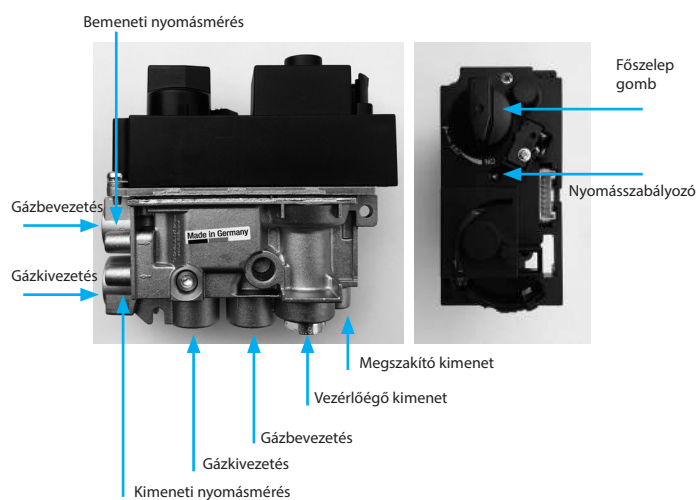
20. ábra GV60 vezérlő alaphelyzetben
