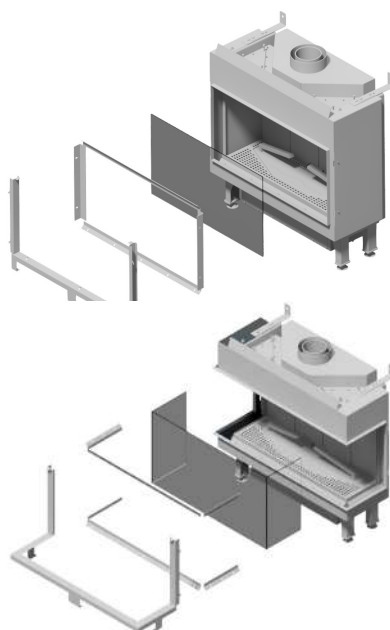
Rys. 18. Sposób demontażu szyby Fig. 18. Method of glass removal Fig. 18. Método de extracción del vidrio Obr. 18. Jak vyjmout sklo Abb. 18: Methode der Glasentfernung Fig. 18. Metodo di rimozione del vetro Рис 18. Способ демонтажа стекла Figur 18. Demontering av glass Figura: 18. Como desmontar o vidro Fig. 18. Cum se demontează sticla Sl. 18. Kako razstaviti steklo Fig. 18. Hur man demonterar glaset
