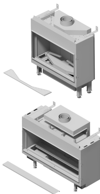
Rys. 19. Sposób demontażu elementu rewizyjnego Fig. 19. Method of dismantling the inspection element Fig. 19. Método de desmontaje del elemento de inspección Obr. 19. Způsob demontáže kontrolního prvku Abb. 19: Verfahren zur Demontage des Inspektionselements Fig. 19. Metodo di smontaggio dell'elemento d'ispezione Рис 19. Способ демонтажа ревизионного элемента Figur 19. Metode for å demontere revisjon element Fig. 19: Méthode de démontage de l'élément d'inspection Obr. 19. Spôsob demontáže revízneho prvku Kuva 19. Menetelmä tarkistuselementin purkamiseksi ábra 19. Az ellenőrző elem szétszerelése Fig. 19. Metode til afmontering af inspektionselementet
