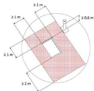
A - B Střešní okno
