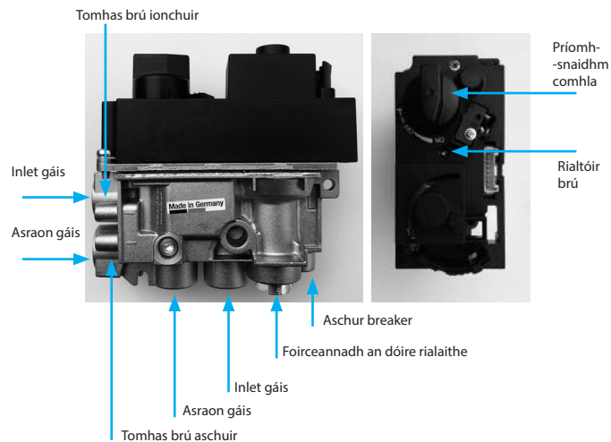
Fíor 20. Rialaitheoir GV60 sa suíomh bunúsach
