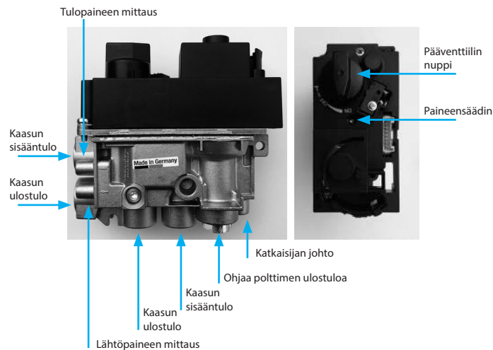
Kuva 20. GV60-ohjain perusasennossa
