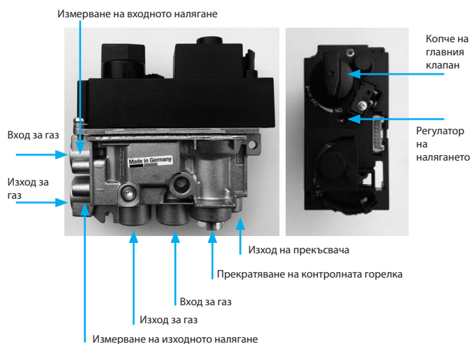
Фиг. 20. Контролер GV60 в основно положение
