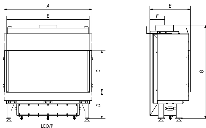
Rys. 2. Wymiary wkładów gazowych z serii LEO
