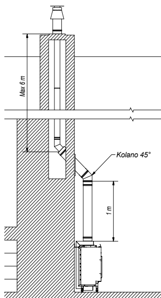
Rys. 10. Sposób instalacji urządzenia z użyciem istniejącego komina
