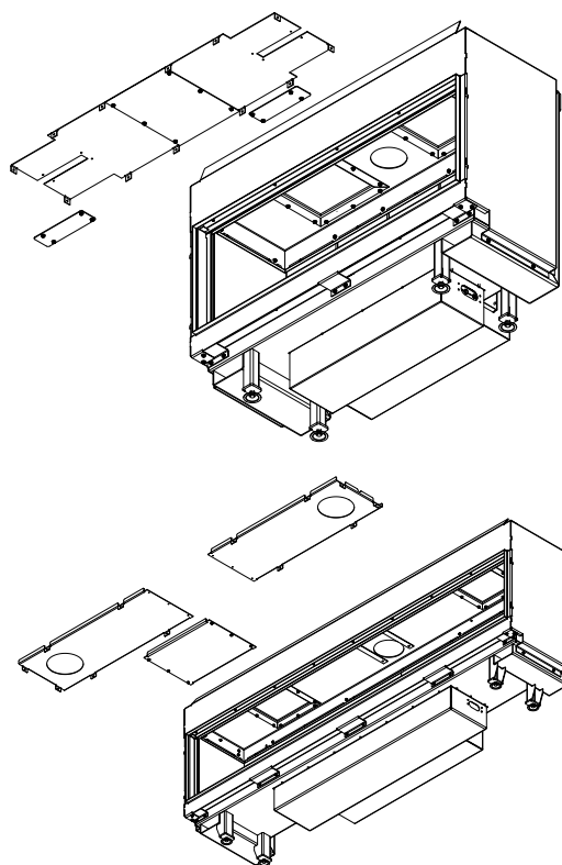
Rys. 13. Demontaż deflektorów LEO100 i LEO200 Fig. 13. Dismantling LEO100 and LEO200 deflectors Fig. 13. Desmontaje de los deflectores LEO100 y LEO200 Obr. 13. Demontáž deflektorů LEO100 a LEO200 Abb. 13: Demontage der Deflektoren LEO100 und LEO200 Fig. 13. Smontaggio dei deflettori LEO100 e LEO200
